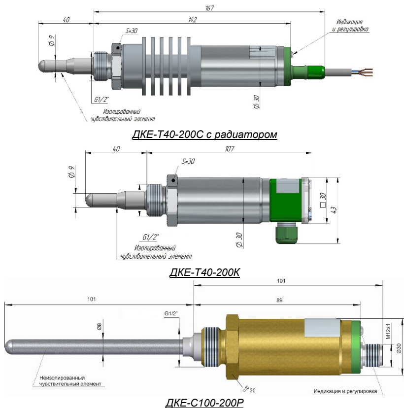
Рисунок 1 - Внешний вид и габаритные размеры (Влагозащитное уплотнение штуцера не показано)
