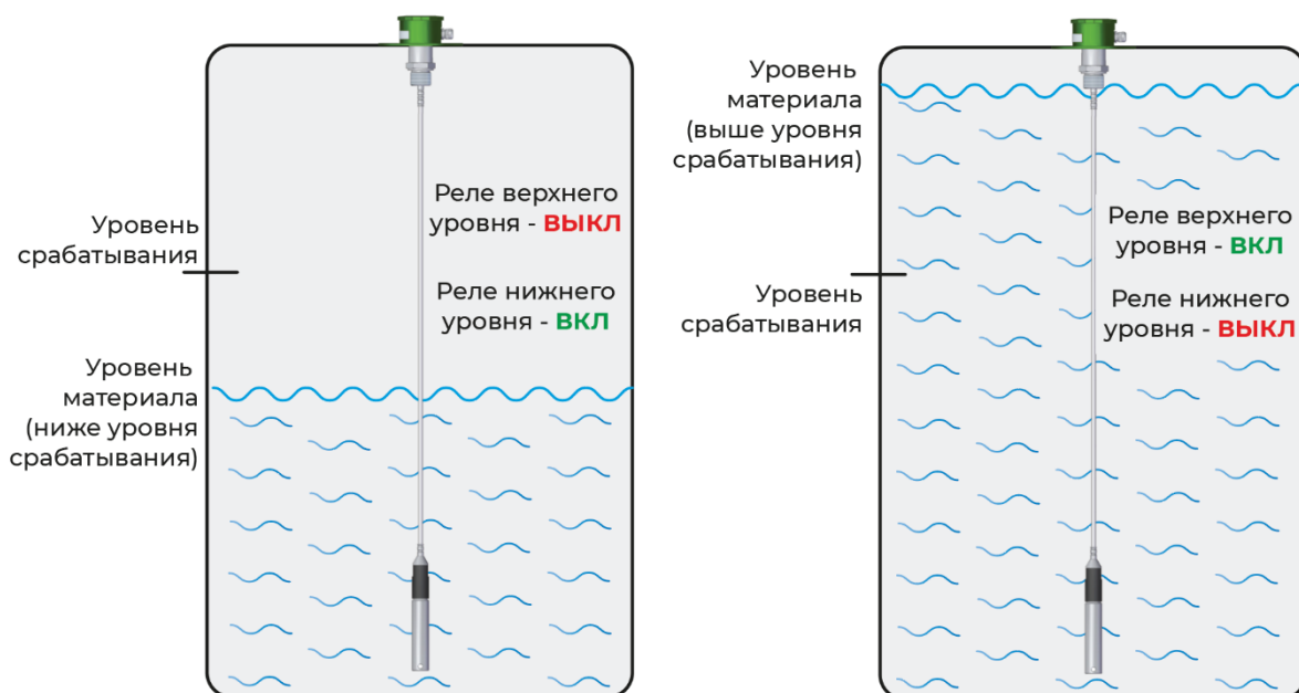
Рис.6 – Состояние реле P \uparrow и P \downarrow в однопороговом режиме
