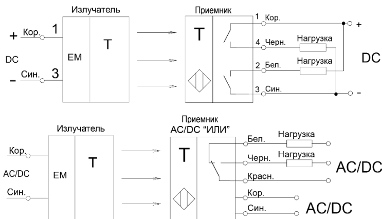
Рисунок 3 - Варианты схем подключения выключателей (цифрами указаны номера контактов разъема)
