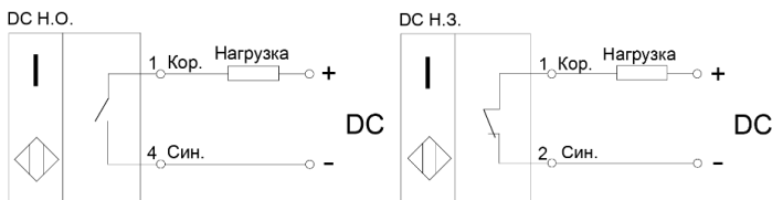
Рисунок 1 - Варианты схем подключения выключателей (цифрами указаны номера контактов разъема или клеммной коробки)
