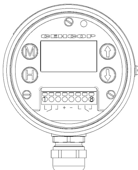
Рисунок 1а – Вид датчика изнутри
