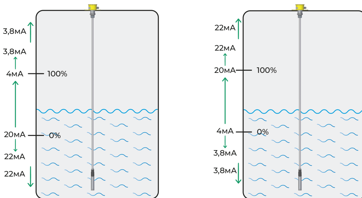
Рис. 10 – Значения выходного тока в режиме 4-20мА за пределами минимального 0% и максимального 100% уровня
