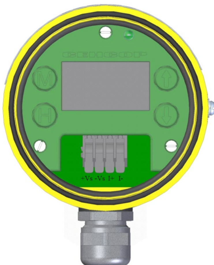
Рисунок 1а – Вид датчика изнутри
