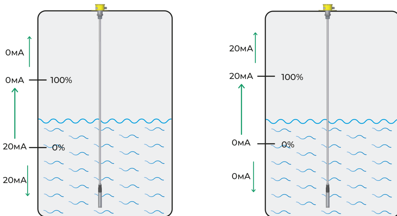
Рис. 11 – Значения выходного тока в режиме 0-20мА за пределами минимального 0% и максимального 100% уровня
