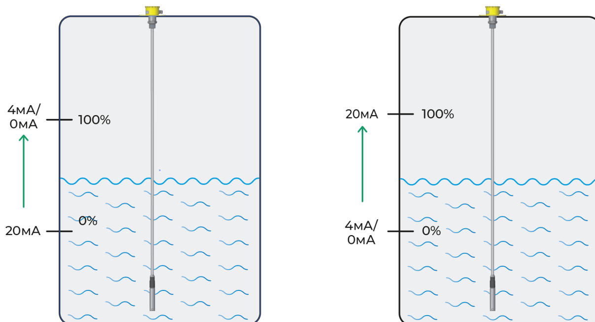
Рис. 7 –направление изменения токового выхода
