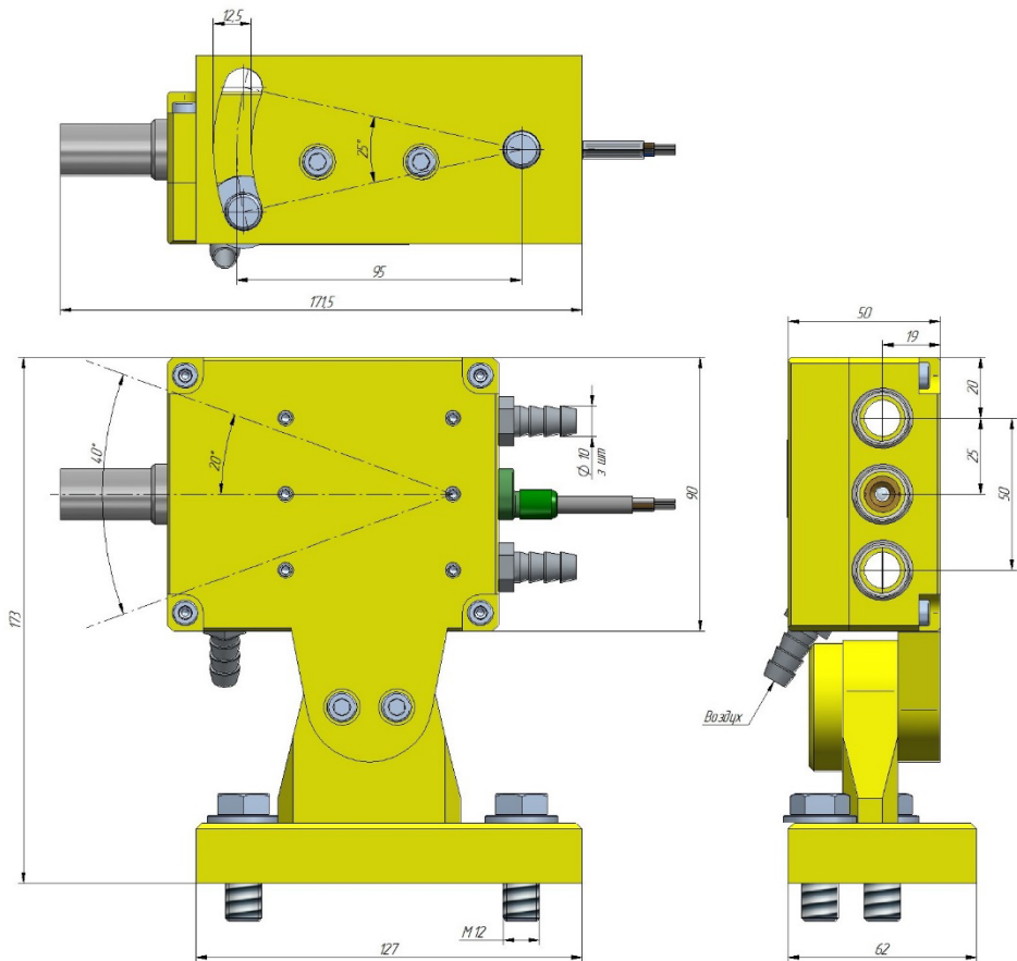
Рисунок 1 - Внешний вид и габаритные размеры детектора
