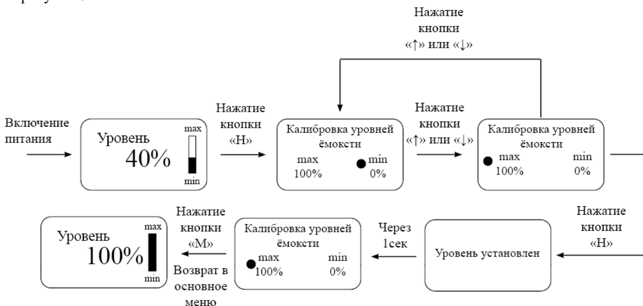
Рис. 6 – программирование максимального (100%) уровня
