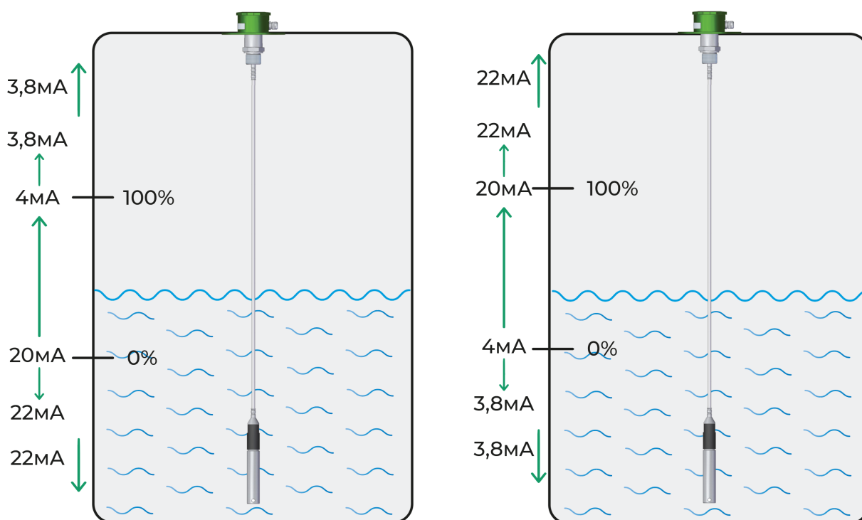
Рис. 10 – Значения выходного тока в режиме 4-20мА за пределами минимального 0% и максимального 100% уровня
