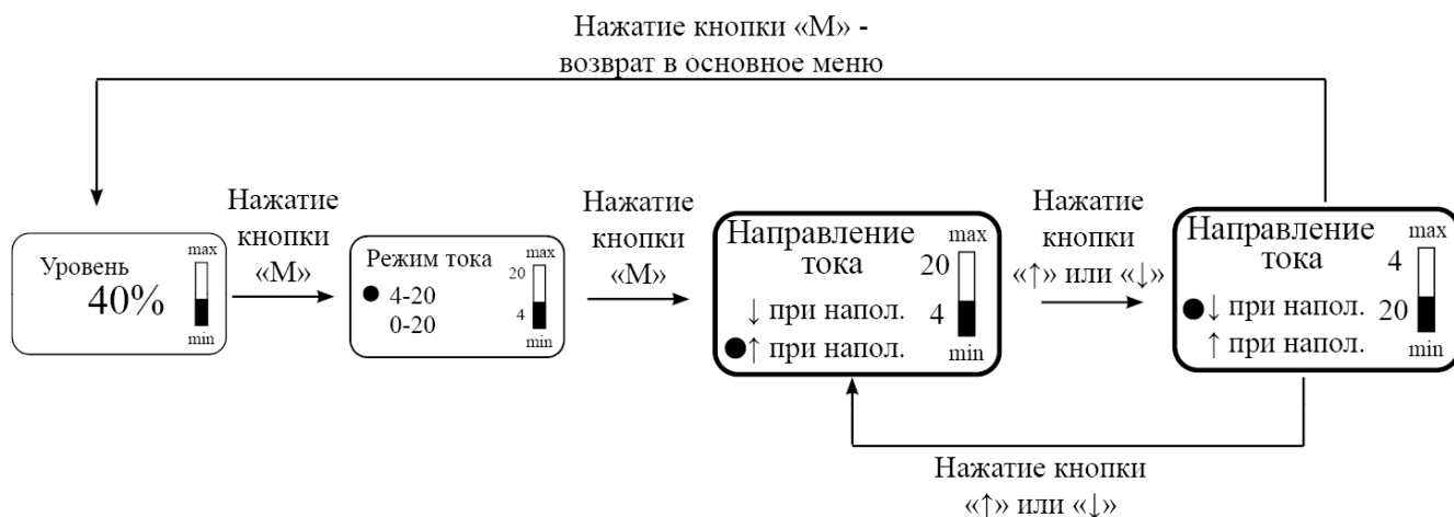
Рис. 8 – выбор направления изменения токового выхода
