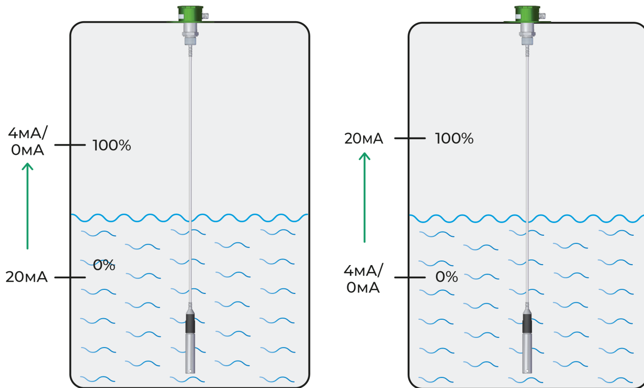
Рис. 7 –направление изменения токового выхода
