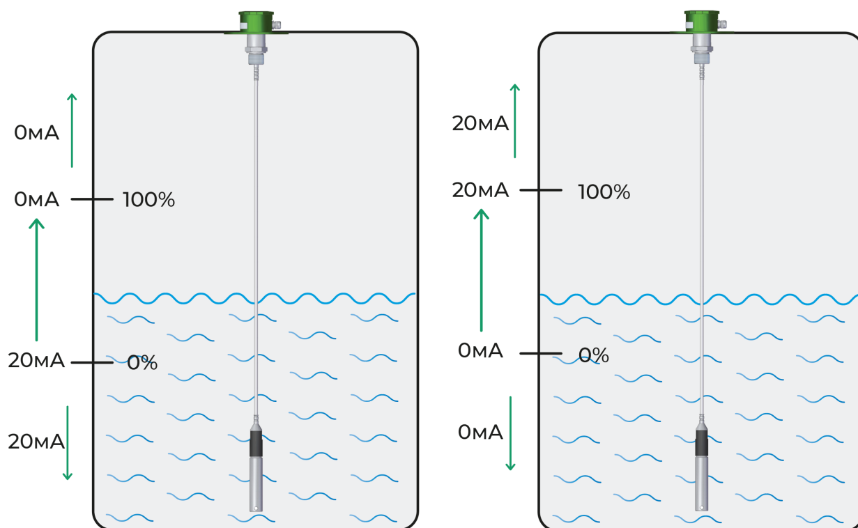
Рис. 11 – Значения выходного тока в режиме 0-20мА за пределами минимального 0% и максимального 100% уровня
