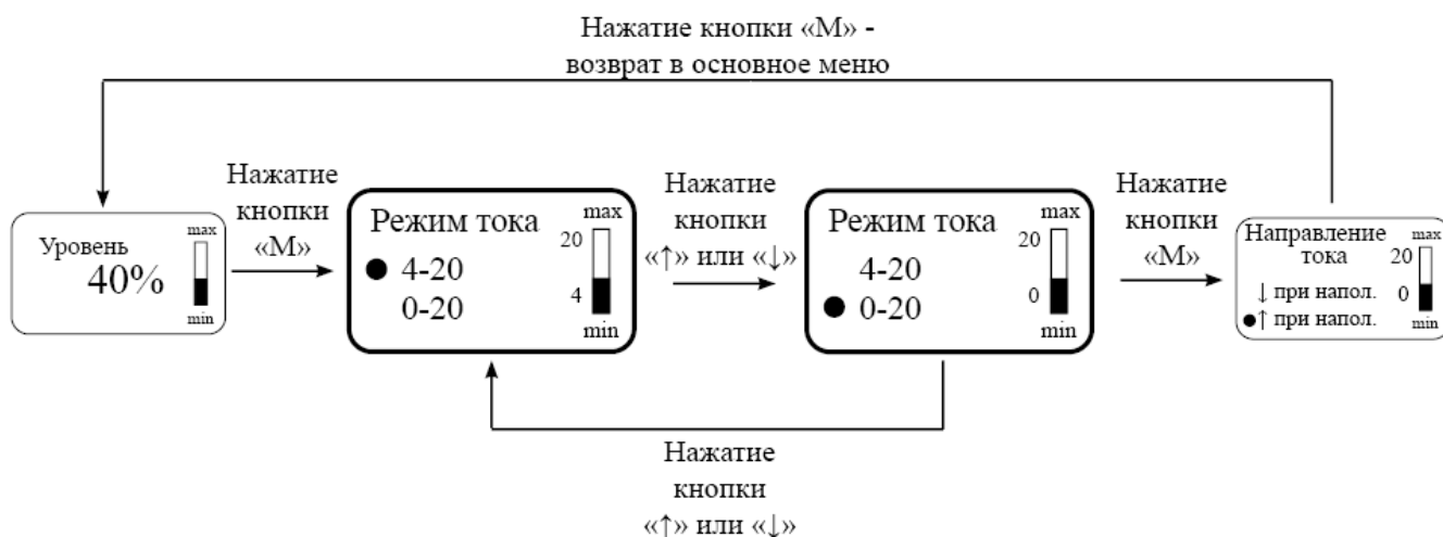
Рис. 9 – выбор диапазона изменения токового выхода
