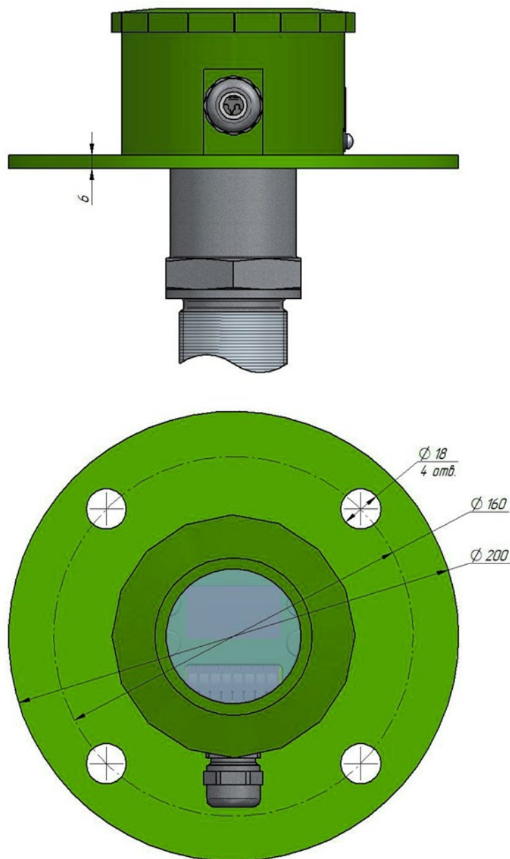
Рис. 3 – фланцевое крепление датчика ДНЕ
