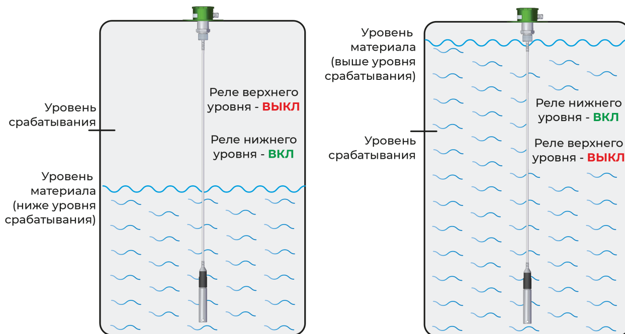
Рис.7 – Состояние реле P↑ и P↓ в однопороговом режиме
