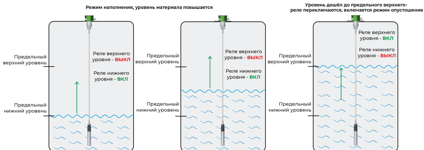
Рис.12 – Состояние реле в режиме наполнение резервуара при наполнении ёмкости.
