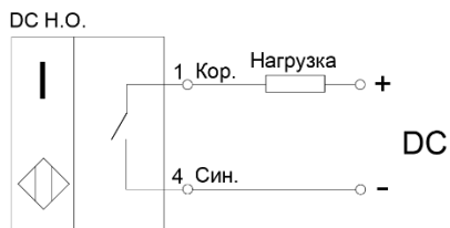
Рисунок 1 - Варианты схем подключения выключателей (цифрами указаны номера контактов)
