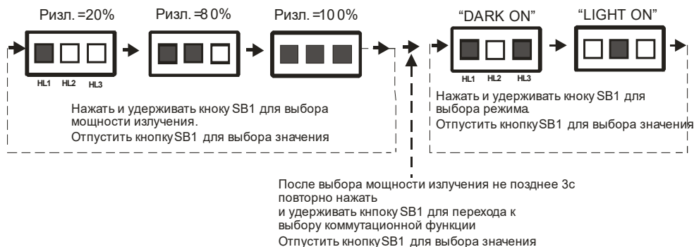
Рисунок 4 - Работа индикаторов при настройке выключателей
