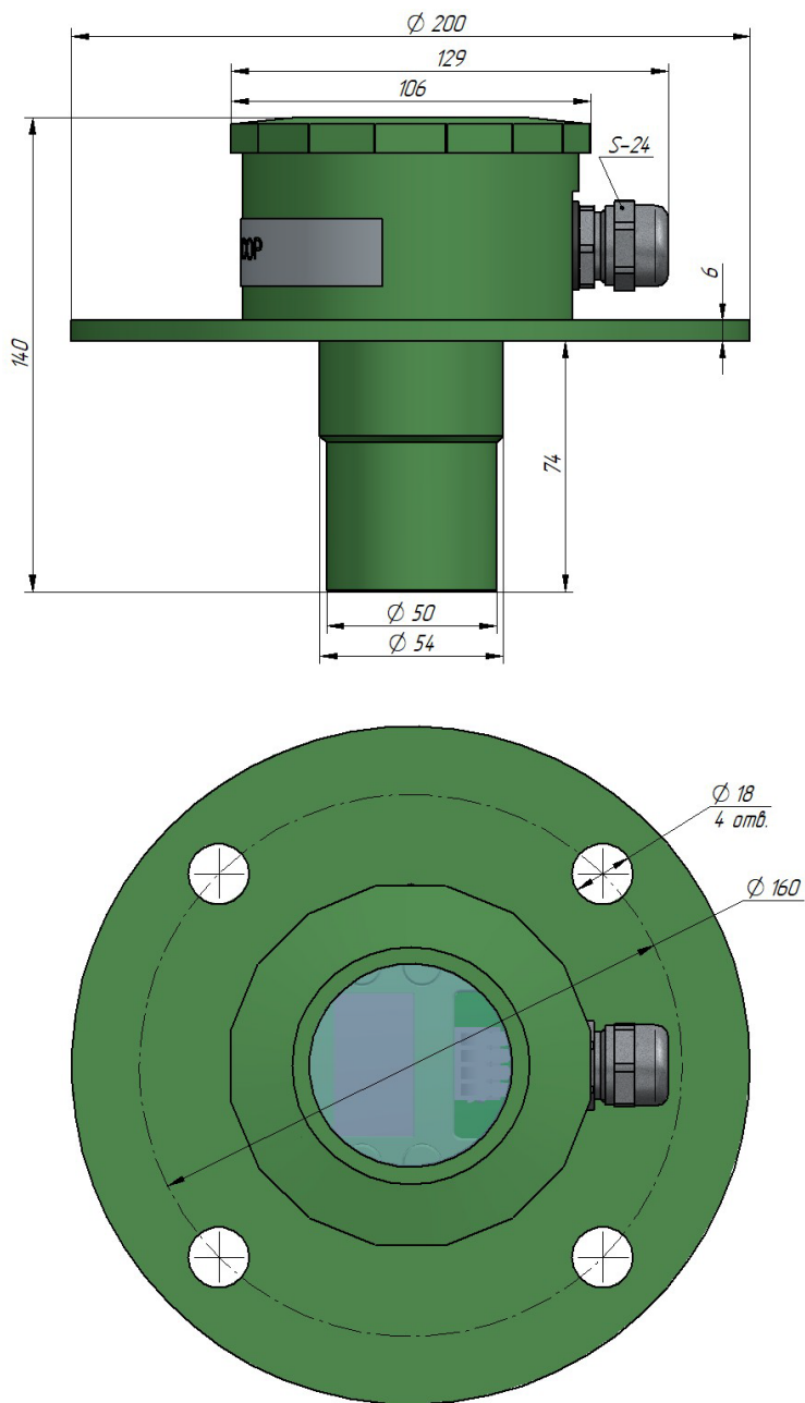
Рисунок 1 – Внешний вид датчика
