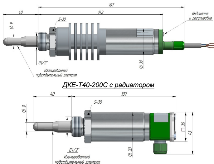
ДКЕ-Т40-200К Рисунок 1 - Внешний вид и габаритные размеры (Влагозащитное уплотнение штуцера не показано)
