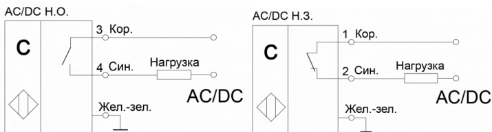
Рисунок 2 - Варианты схем подключения датчиков
