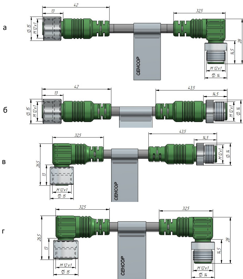
Рисунок 2 - Внешний вид и габаритные размеры соединительных кабелей с двумя разъемами: а) ПР-УВ, б) ПР-ПВ, в) УР-ПВ, г) УР-УВ П – прямой, В – угловой, Р – розетка, В – вилка
