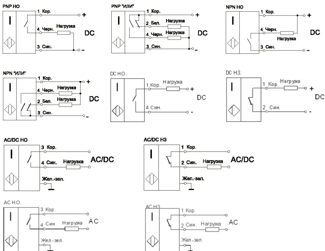
Рисунок 1 - Варианты схем подключения датчиков
