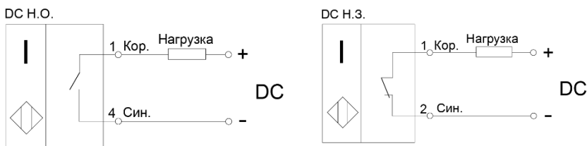
Рисунок 1 - Варианты схем подключения выключателей (цифрами указаны номера контактов разъема)
