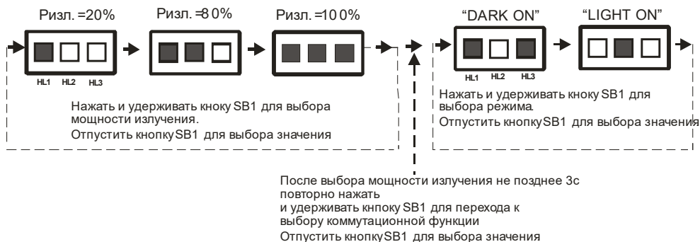
Рисунок 4 - Работа индикаторов при настройке выключателей
