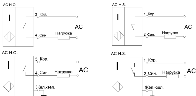
Рисунок 1 - Варианты схем подключения выключателей (цифрами указаны номера контактов клеммной коробки)
