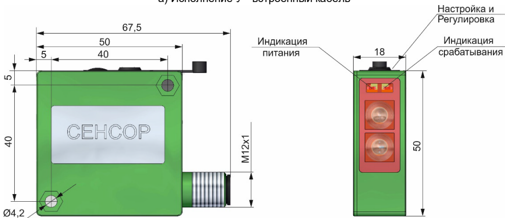
б) Исполнение Р - разъем М12 на корпусе
