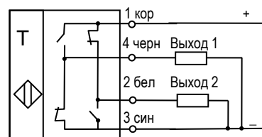
Рис. 4. Приемник Выход 1 – PNP, НО Выход 2 – PNP, НЗ
