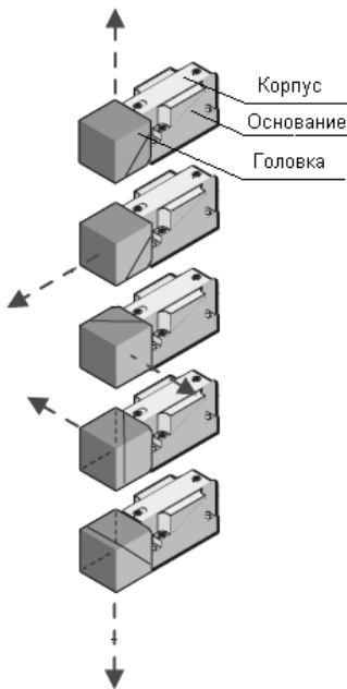
Рисунок 2 - Варианты установки головки
