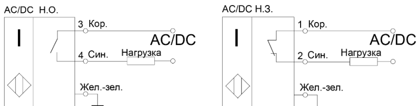
Рисунок 1 - Варианты схем подключения выключателей (цифрами указаны номера контактов)
