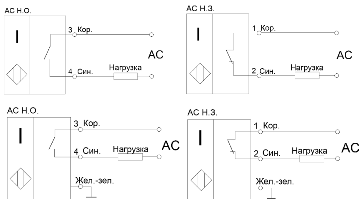
Рисунок 1 - Варианты схем подключения выключателей (цифрами указаны номера контактов)
