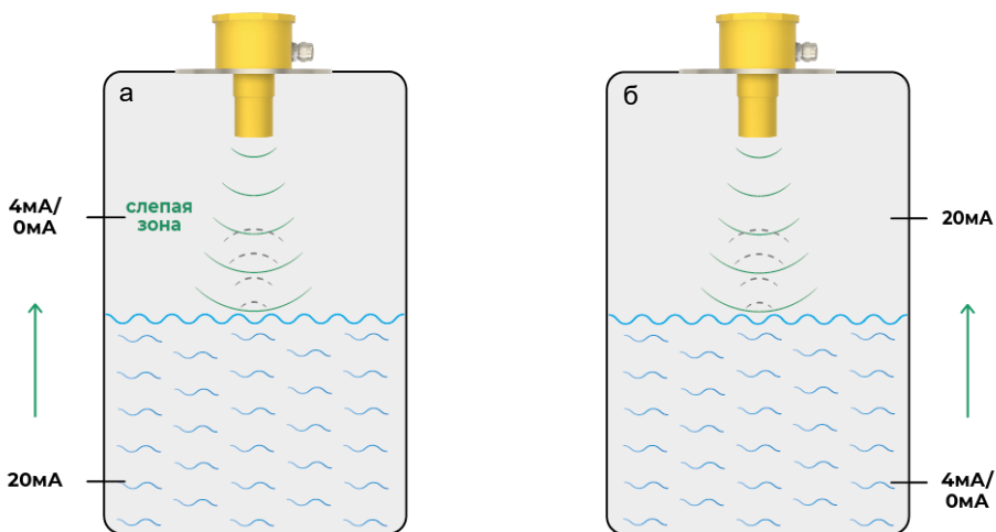
Рисунок 4 – Изменение тока аналогового выхода при наполнении (а – уменьшение, б – увеличение)
