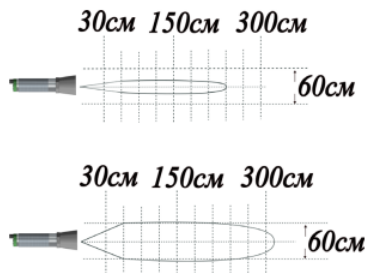
Рисунок 13 – Диаграмма направленности ДПУ-М30-100У-3110-СА для небольших объектов (25x25мм) и крупных объектов (250x250мм)
