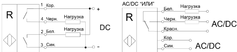
Рисунок 3 - Варианты схем подключения выключателей (цифрами указаны номера контактов разъема)
