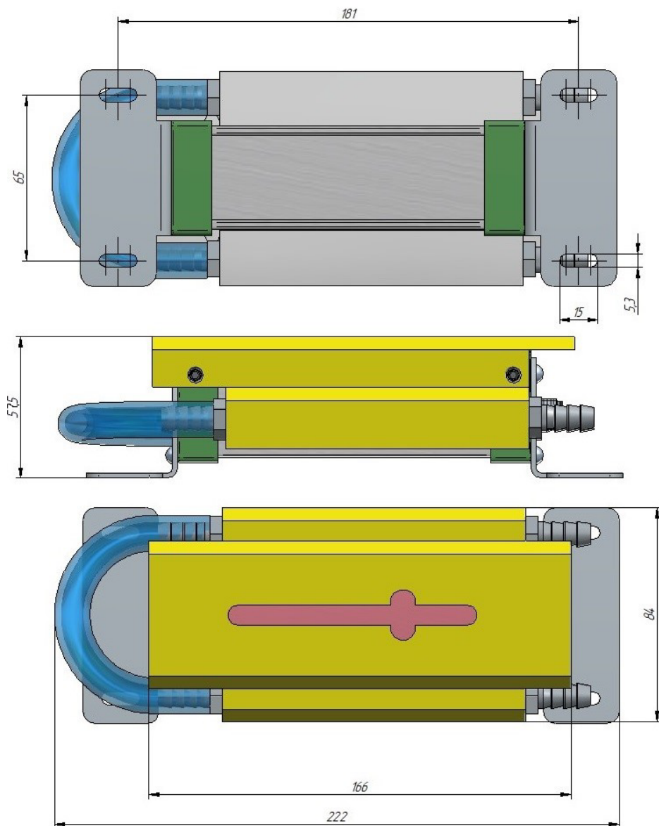
Рисунок 1 - Внешний вид и габаритные размеры барьеров
