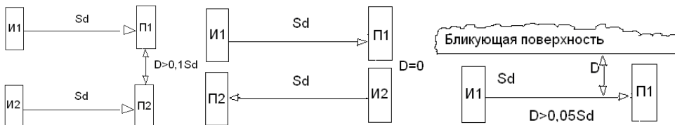
Рисунок 3 - Варианты установки барьеров И - излучатель; П – приёмник; Sd – зона чувствительности.
