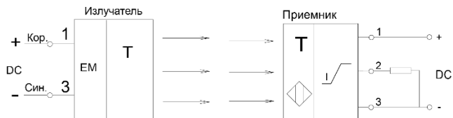
Рисунок 2 - Варианты схем подключения
