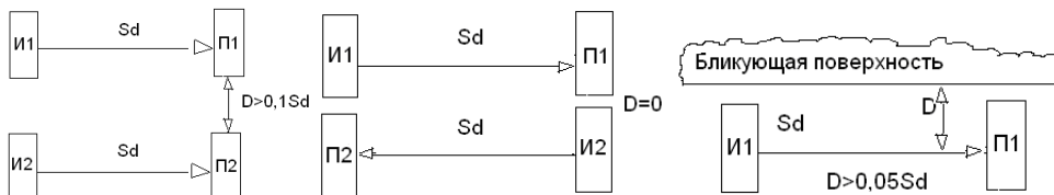
Рисунок 4 - Варианты установки ДПО-ЭК20
