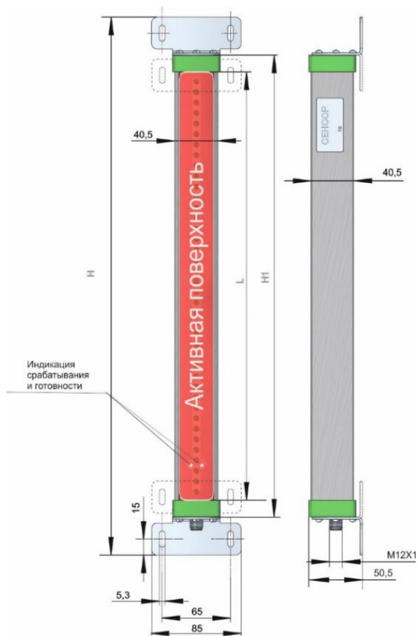
Рисунок 1 - Внешний вид и габаритные размеры Размер H=(L+104) мм; H1=(L+32) мм
