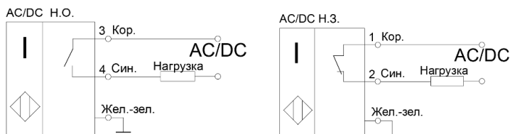
Рисунок 1 - Варианты схем подключения выключателей
