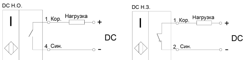
Рисунок 1 - Варианты схем подключения выключателей
