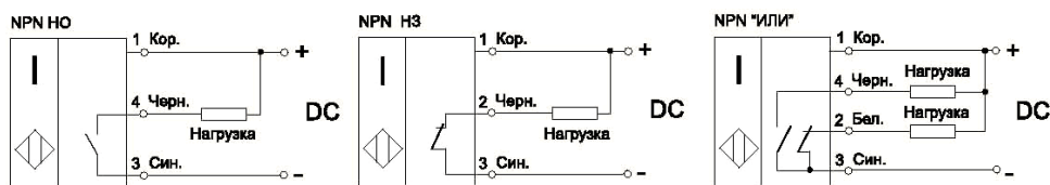
Рисунок 1 - Варианты схем подключения датчиков
