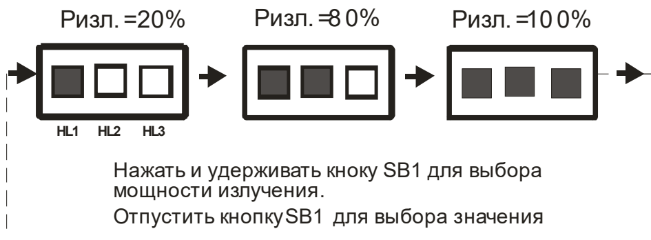
Рисунок 4 - Работа индикаторов в режиме выбора мощности излучения
