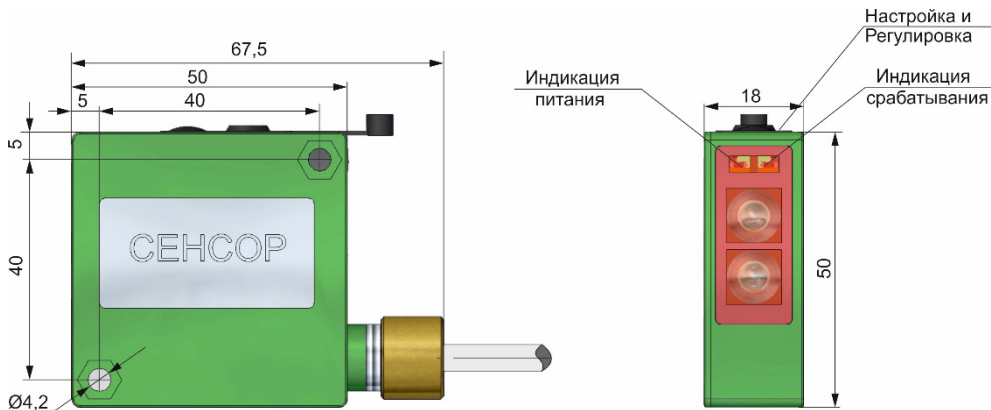
а) Исполнение У - встроенный кабель
