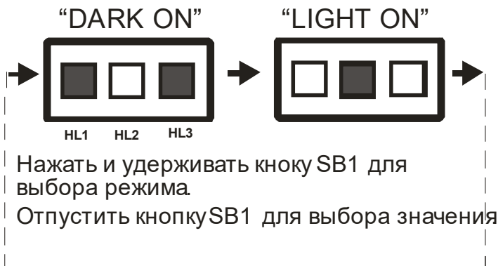
Рисунок 5 - Работа индикаторов в режиме выбора коммутационной функции
