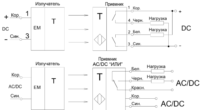
Рисунок 3 - Варианты схем подключения выключателей (цифрами указаны номера контактов разъема)
