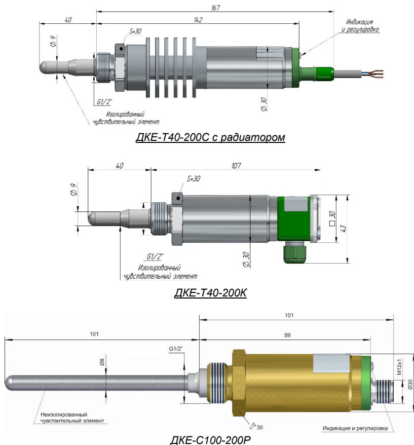
Рисунок 1 - Внешний вид и габаритные размеры (Влагозащитное уплотнение штуцера не показано)
