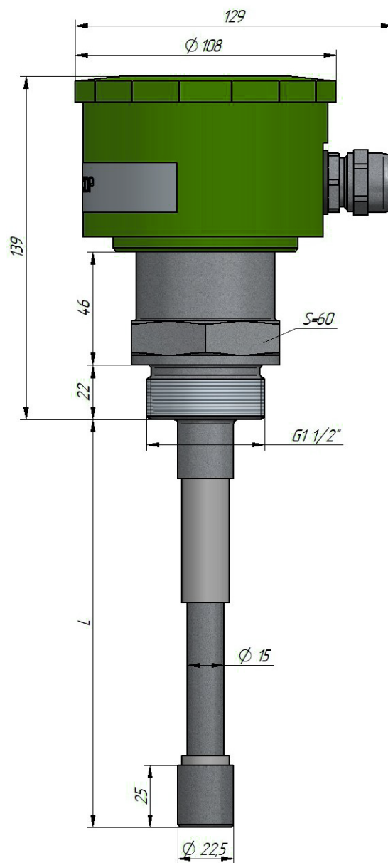
ДНЕ-хС(002...-020)-110Кх0 Рис. 1д. Жесткий неизолированный ЧЭ типа «С» без радиатора
