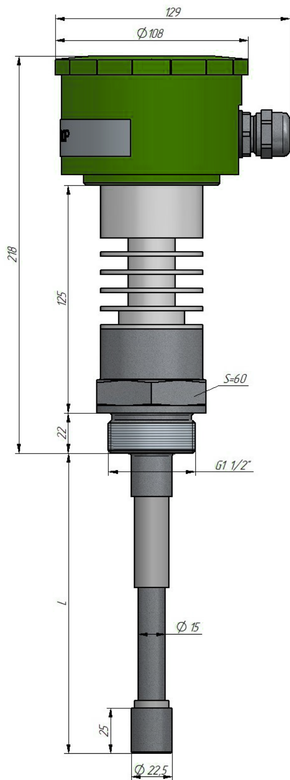
ДНЕ-хС(002...020)-110Тх0 Рис. 1г. Жесткий неизолированный ЧЭ типа «С» с радиатором
