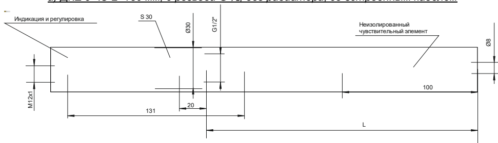
б) ДКЕ с ЧЗ от 200 до 500 мм, с резьбой G 1/2, без радиатора, с разъемом
