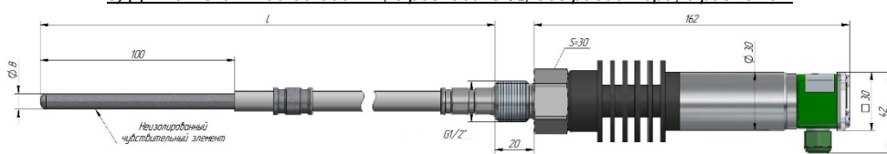
в) ДКЕ с ЧЗ от 200 до 500 мм, с резьбой G 1/2, с радиатором, с клеммником
