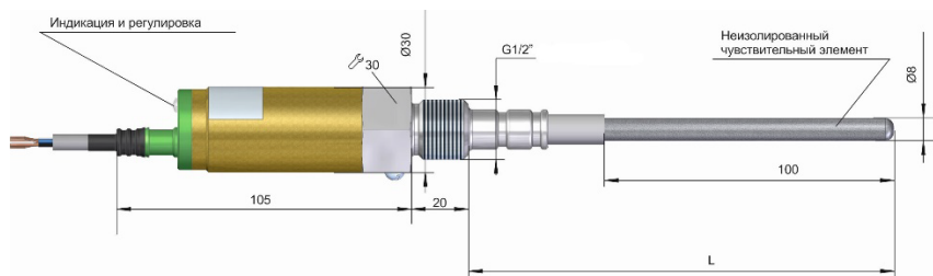
а) ДКЕ с ЧЗ L=150 мм, с резьбой G 1/2, без радиатора, со встроенным кабелем
