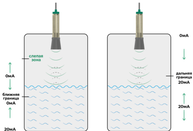
Рисунок 7 – Значения выходного тока в режиме 0-20mA за ближней или дальней границами, режим - увеличение тока при удалении материала
