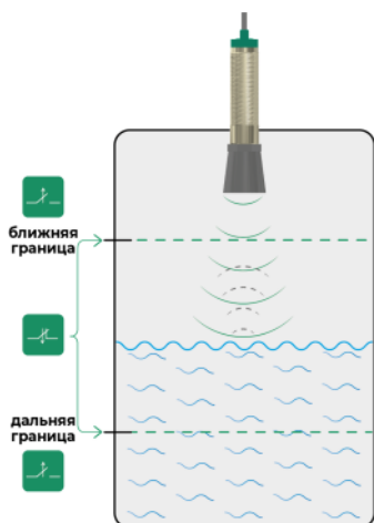
Рисунок 10 – Состояние дискретного выхода в режиме «НО»
