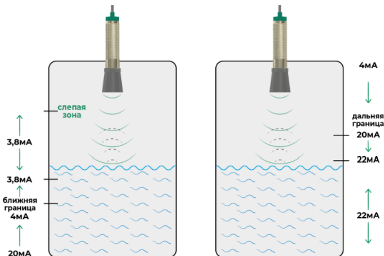
Рисунок 6 - Значения выходного тока в режиме 4-20мА за ближней или дальней границами, режим - увеличение тока при удалении материала
