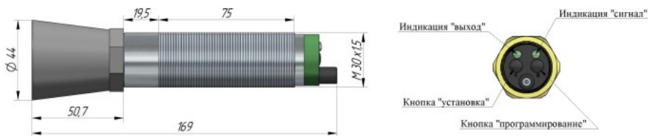
Рисунок 1 – Внешний вид и органы управления ДПУ
