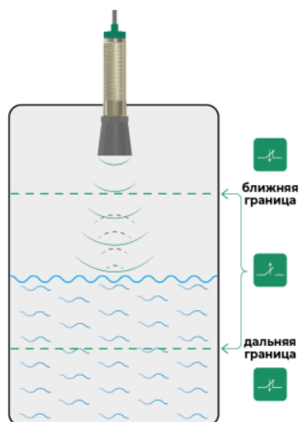
Рисунок 11 – Состояние дискретного выхода в режиме «НЗ»
