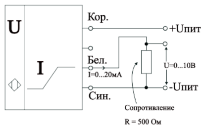
Рисунок 9 - Преобразование токового сигнала в сигнал по напряжению
