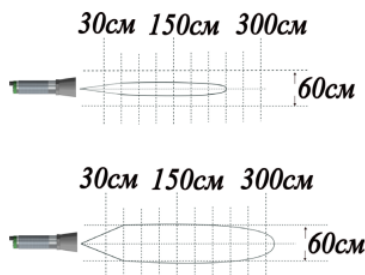
Рисунок 13 – Диаграмма направленности ДПУ-М30-100У-3110-СА для небольших объектов (25х25мм) и крупных объектов (250х250мм)
