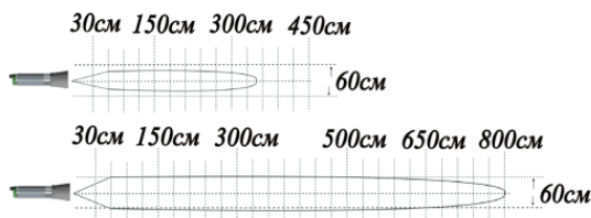
Рисунок 15 – Зона обнаружения ДПУ-М30-100У-8110-СА для небольших объектов (25х25мм) и крупных объектов (250х250мм)
