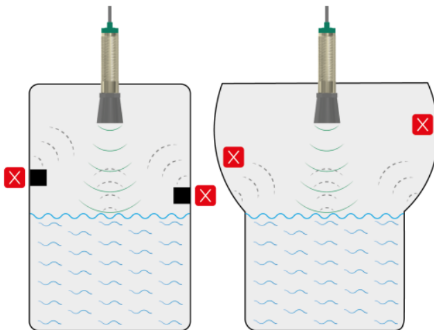
Рисунок 16 – Обнаружение датчиков сторонних/нежелательных объектов
