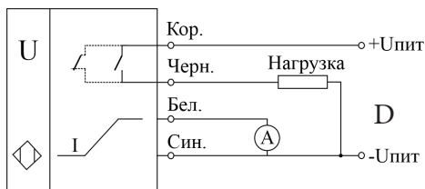
Рисунок 2 - Схема подключения
