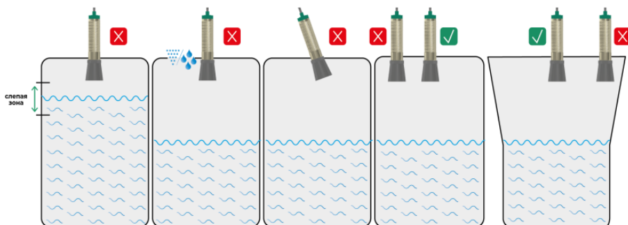
Рисунок 12 – Правила установки ДПУ
