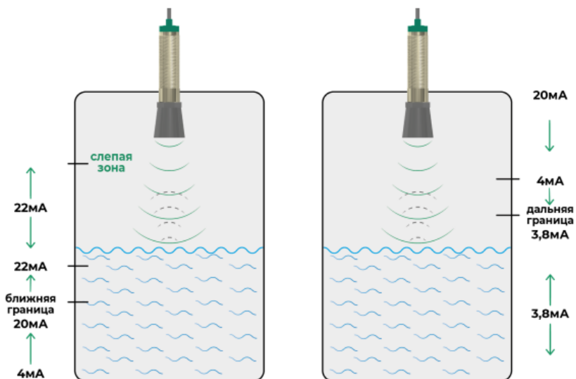
Рисунок 5 - Увеличение тока аналогового выхода при приближении объекта
