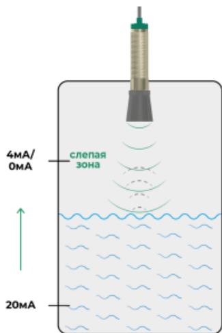
Рисунок 3 – Увеличение тока аналогового выхода при удалении
