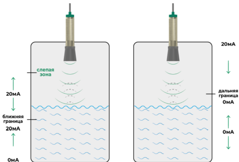
Рисунок 8 – Значения выходного тока в режиме 0-20mA за ближней или дальней границами, режим - увеличение тока при приближении материала
