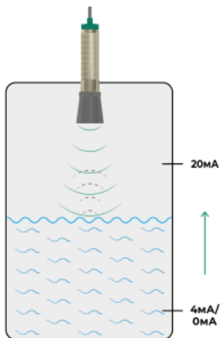
Рисунок 4 – Увеличение тока аналогового выхода при приближении
