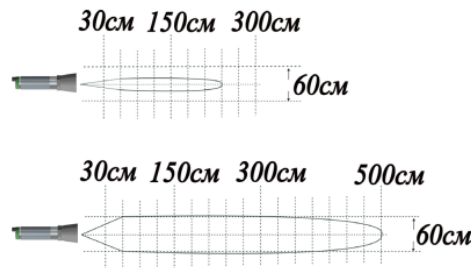
Рисунок 14 – Зона обнаружения ДПУ-М30-100У-5110-СА для небольших объектов (25х25мм) и крупных объектов (250х250мм)
