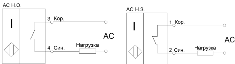
Рисунок 1 - Варианты схем подключения выключателей
