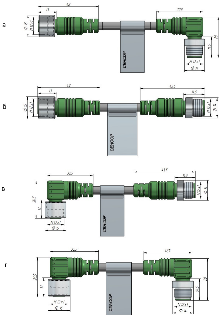
Рисунок 2 - Внешний вид и габаритные размеры соединительных кабелей с двумя разъемами: а) ПР-УВ, б) ПР-ПВ, в) УР-ПВ, г) УР-УВ
