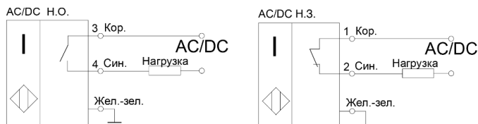
Рисунок 1 - Варианты схем подключения выключателей
