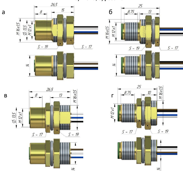
Рисунок 2 - Внешний вид и габаритные размеры блочных разъемов: а) розетка тыловая, б) вилка тыловая, в) розетка фронтная, г) вилка фронтная
