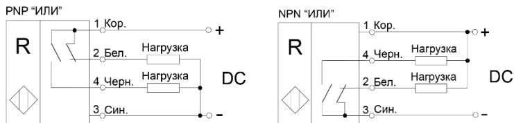
Рисунок 1 - Варианты схем подключения выключателей (цифрами указаны номера контактов)
