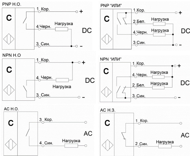
Рисунок 2 - Варианты схем подключения выключателей (цифрами указаны номера контактов клеммной коробки и разъема)
