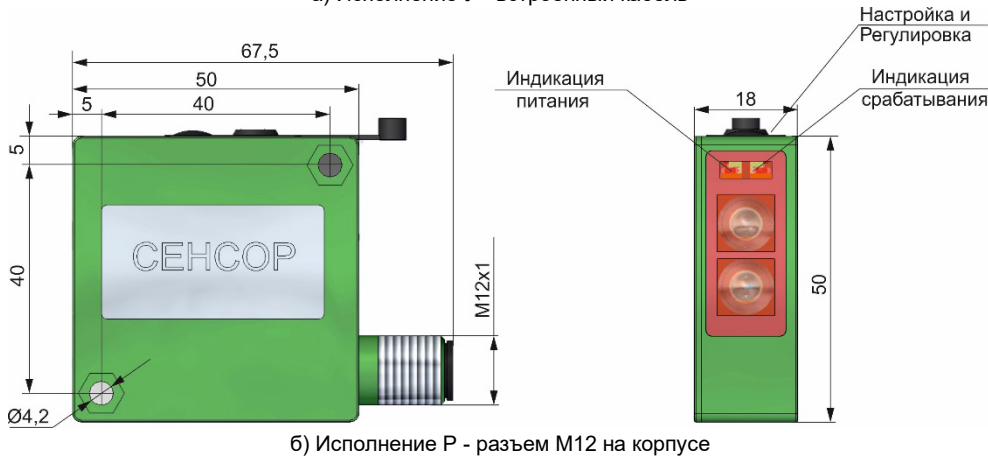
Рисунок 1 – Внешний вид выключателей
