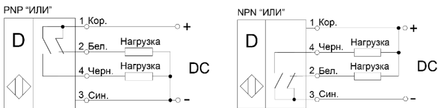
Рисунок 1 - Варианты схем подключения датчиков (цифрами указаны номера контактов разъема)
