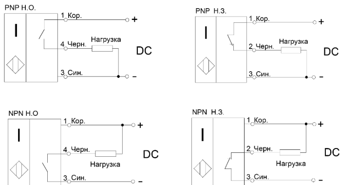
Рисунок 1 - Варианты схем подключения выключателей (цифрами указаны номера контактов разъема)
