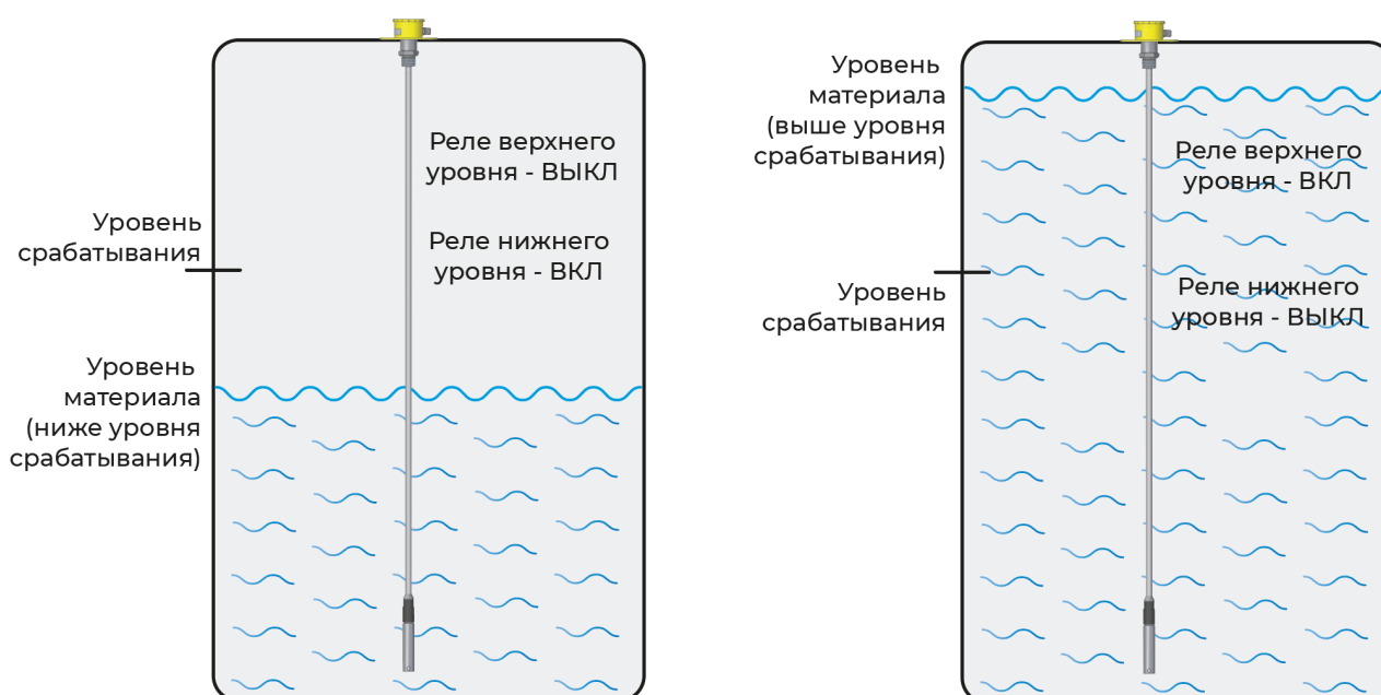
Рис.7 – Состояние реле P\uparrow и P\downarrow в однопороговом режиме
