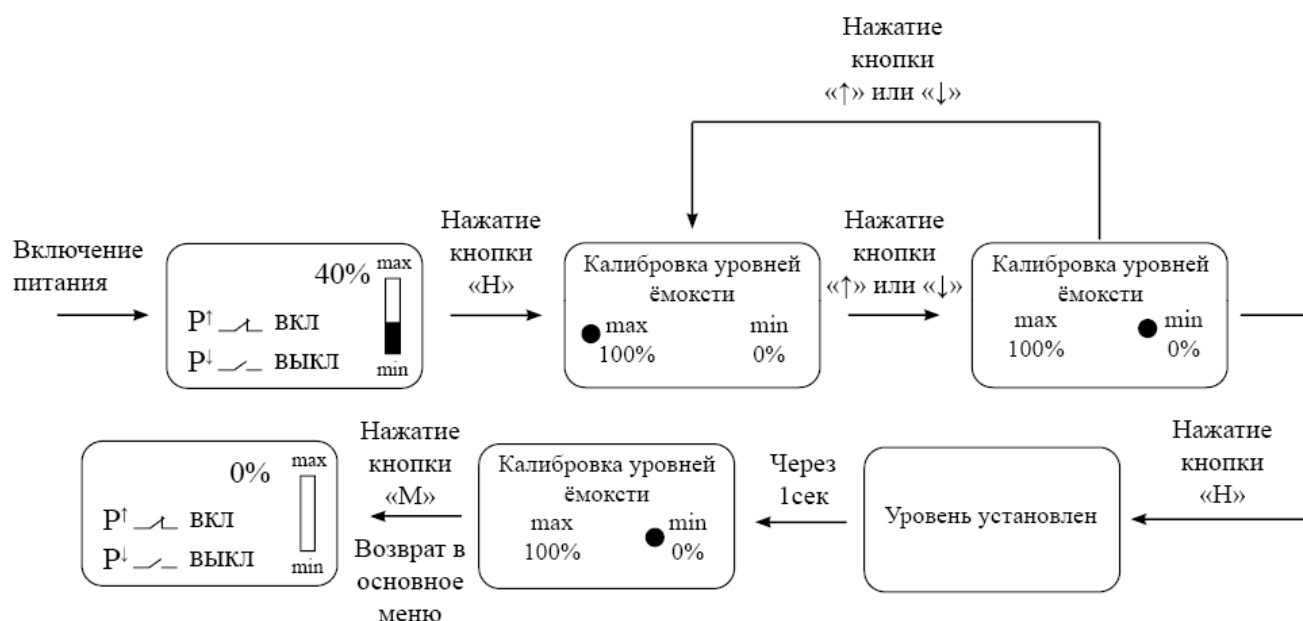
Рис. 5 – программирование минимального (0%) уровня
