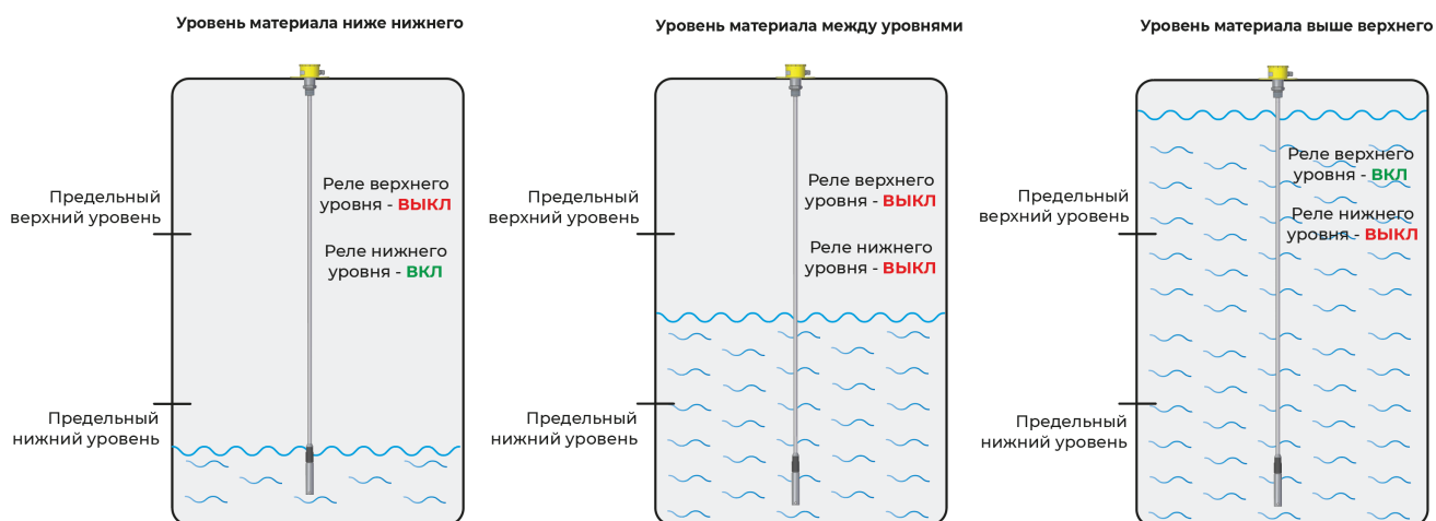
Рис.9 – Состояние реле P\uparrow и P\downarrow в двухпороговом режиме
