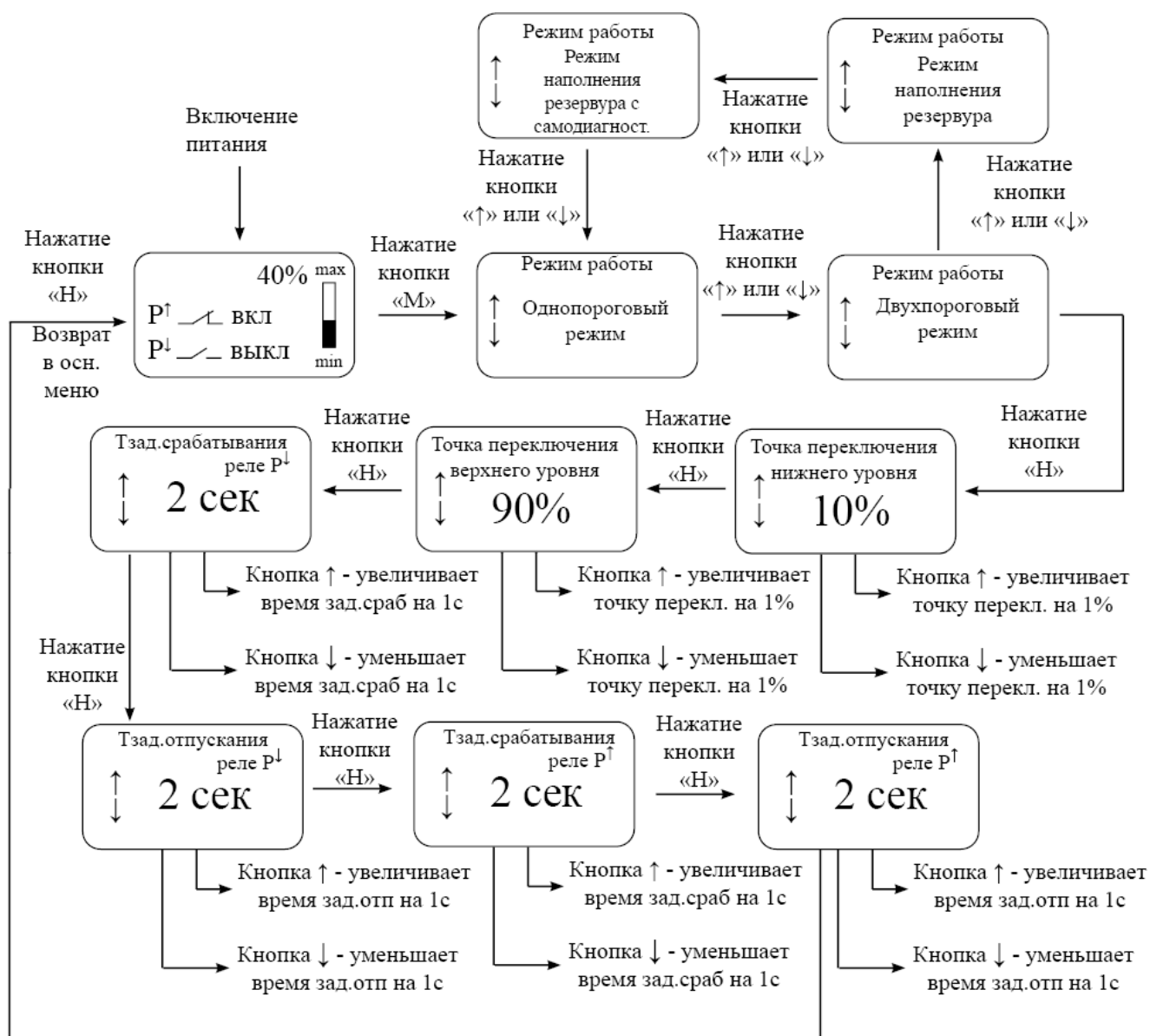
Рис.10 – Выбор и настройка двухпорогового режима работы.
