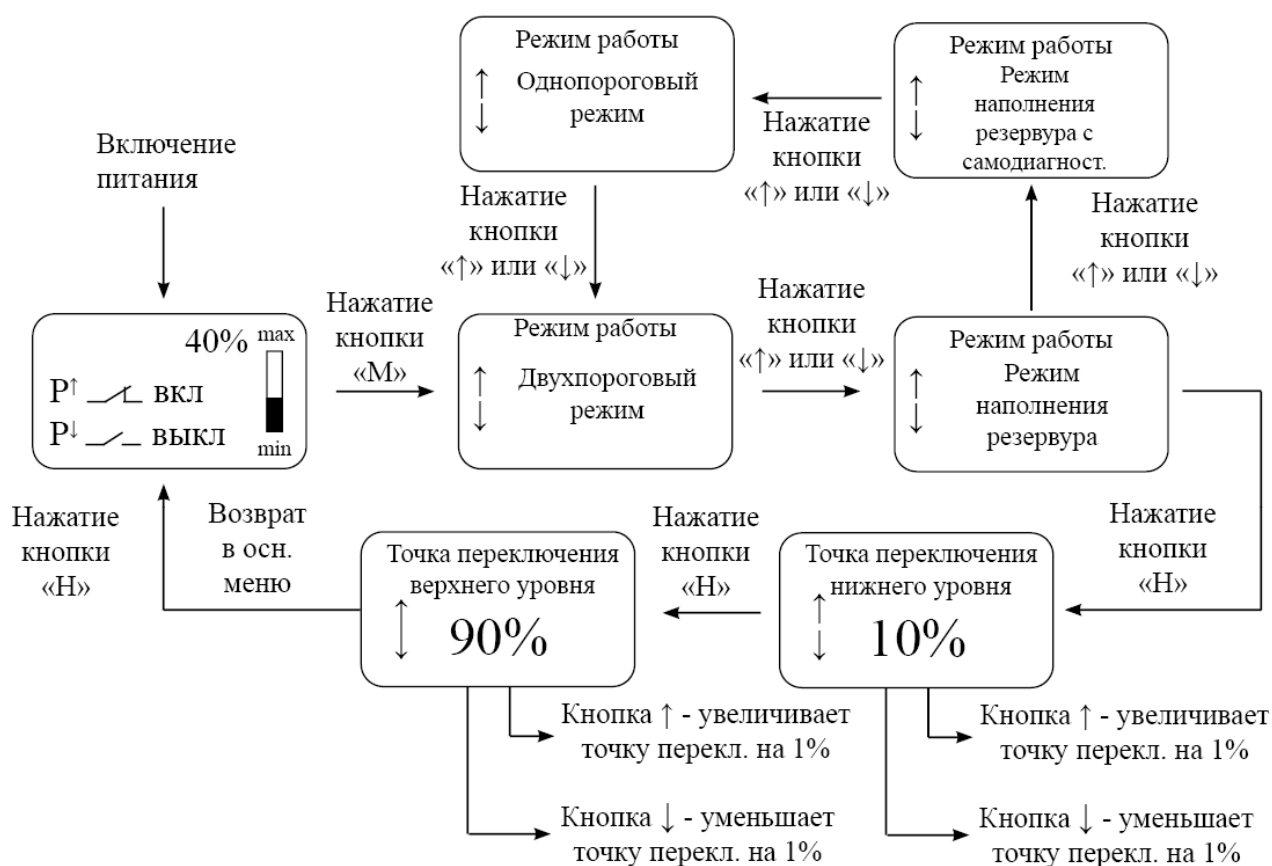
Рис.13 – Выбор и настройка режима наполнения резервуара.
