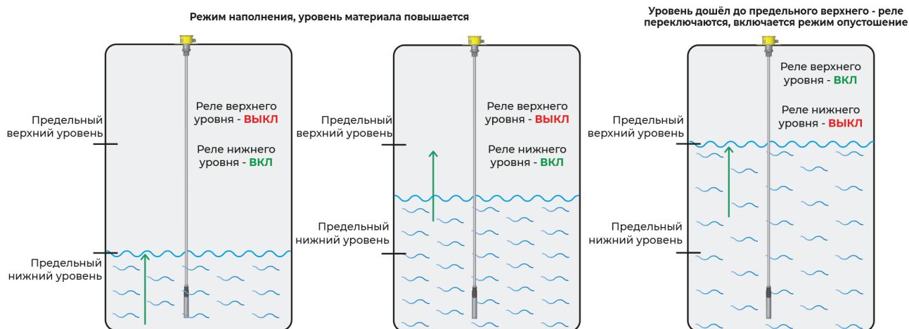
Рис.12 – Состояние реле в режиме наполнение резервуара при наполнении ёмкости.
