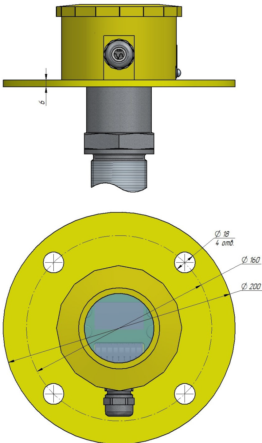
Рис. 3 – фланцевое крепление датчика ДНЕ
