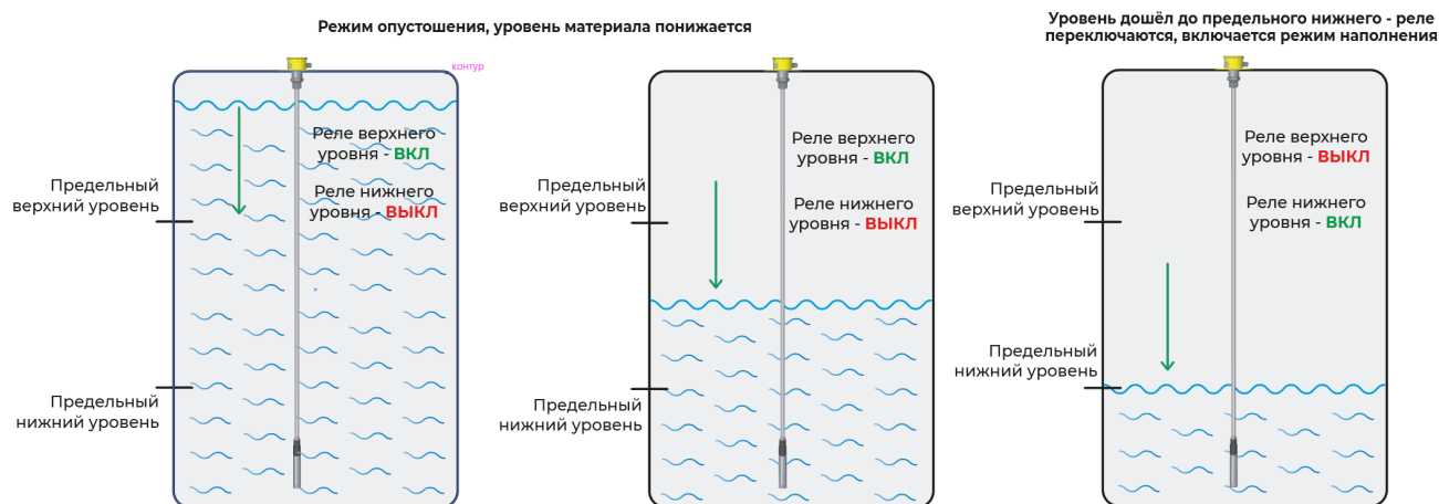
Рис.11 – Состояние реле в режиме наполнение резервуара при опустошении ёмкости.
