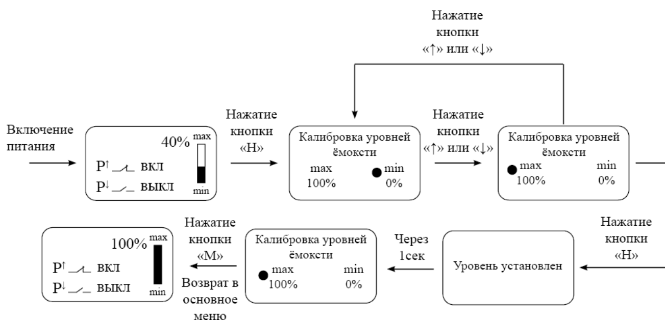
Рис. 6 – программирование максимального (100%) уровня
