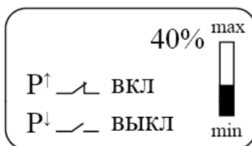
Рис.4 – Основное меню. Отображение информации об уровне заполнения и о состоянии реле
