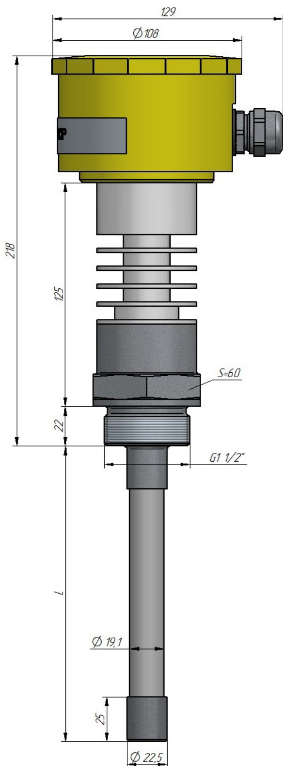
ДНЕ-хТ(002...020)-117Тх0 Рис. 1б. Жесткий изолированный ЧЭ типа «Т» с радиатором
