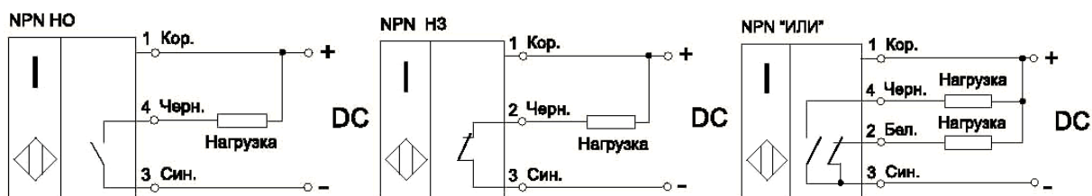
Рисунок 1 - Варианты схем подключения датчиков
