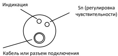
Рисунок 2 – Крышка корпуса у исполнений В, С, Р
