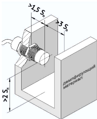
Рисунок 5 – Минимальные расстояния до металлических и демпфирующих объектов при установке неутапленных емкостных выключателей
