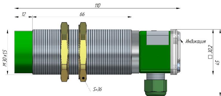
ж) ВБЕ-М30-85К
