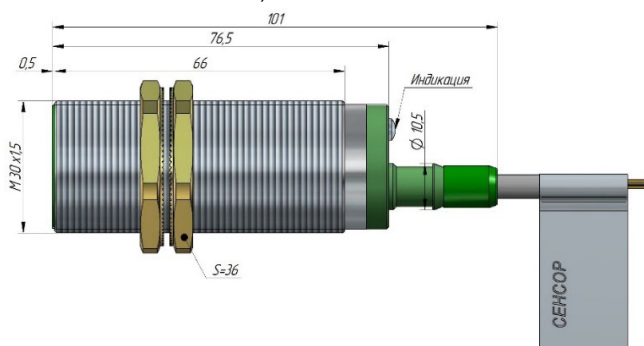
б) ВБЕ-М30-73С
