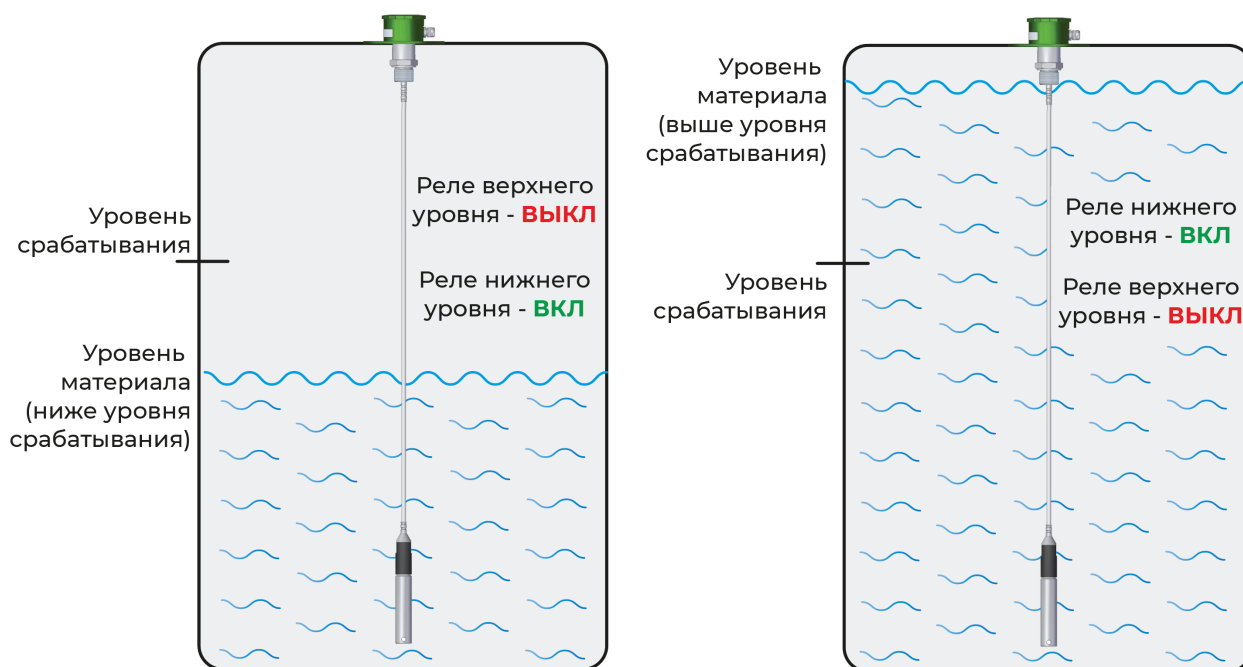
Рис.7 – Состояние реле P↑ и P↓ в однопороговом режиме
