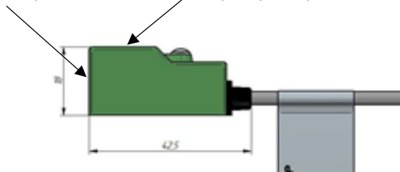
Рисунок 2 – Расположение ЧЭ на примере ВБИ-П18УР
